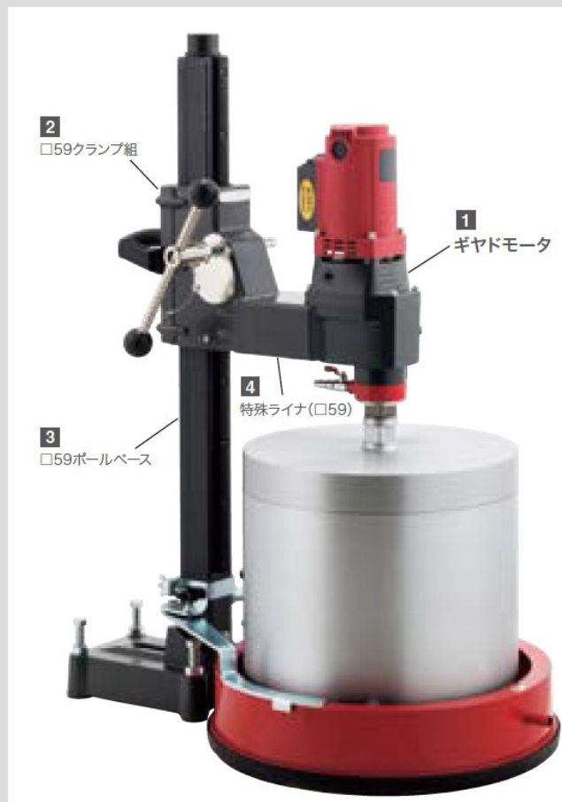
Работа с автоподачей SPM-302i
